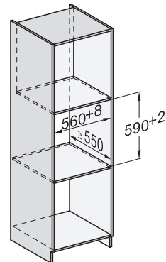
Einbau_DG_DGM_DGC_XL_ESW7x10_EVS7010 Skizze
